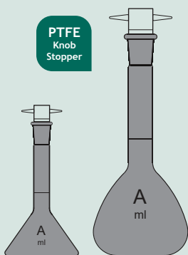
62 AP (5-20 ml) 62 AP (25-2000 ml)
